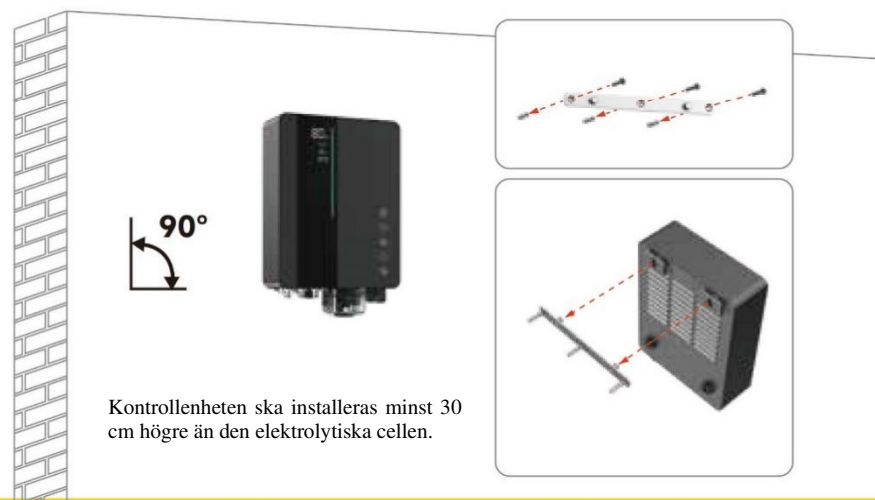
③ Installation av kontrollenhet
