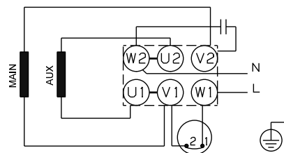
Fig. 15 Tilslutning, 240 V, 1,1 - 2,2 kW
