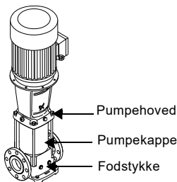
Fig. 17 Varme eller kolde overflader på en CR-, CRI- og CRN-pumpe
