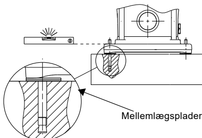
Fig. 6 Oprettning med mellemlægsplader
