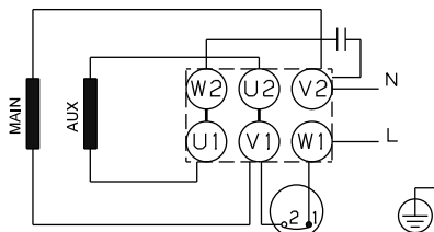
Fig. 14 Tilslutning, 220-230 V, 1,1 - 2,2 kW
