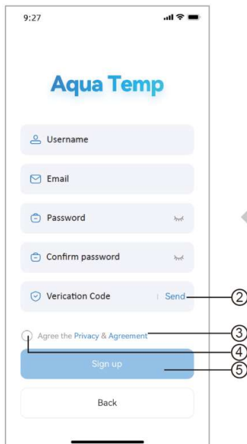
Fig.2 Kontoregistrering-gränssnitt
