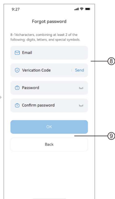
Fig.3 Glömt lösenord-gränssnitt
