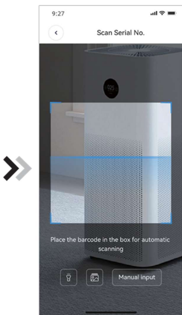
Fig.19 Skanningsgränssnitt
