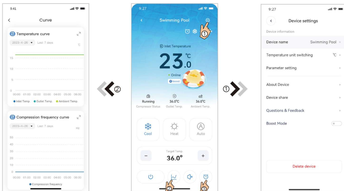
Fig.27 Kurvgränssnitt
