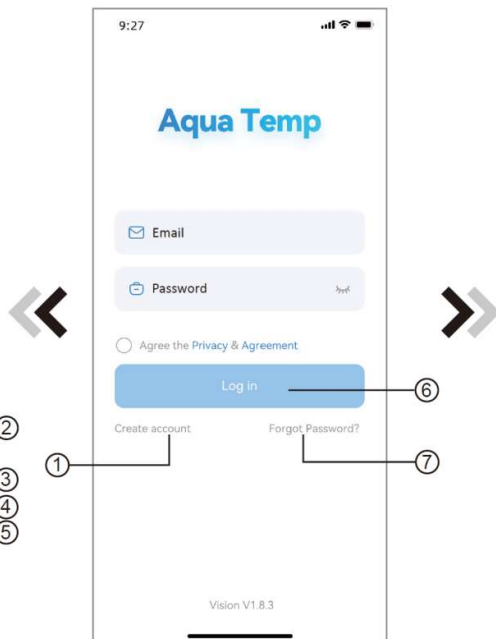
Fig.1 Inloggningsgränssnitt
