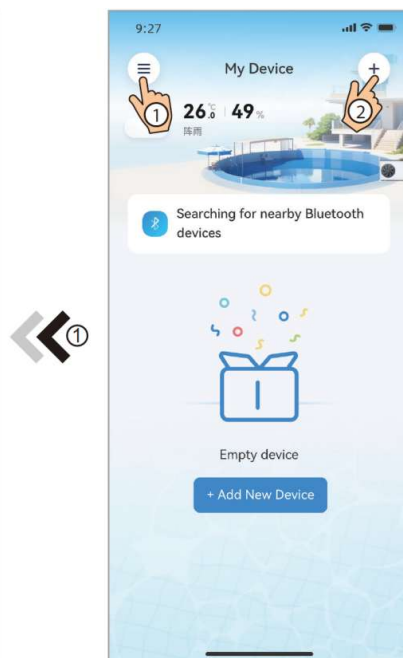
Fig.4 Min enhet-gränssnitt
