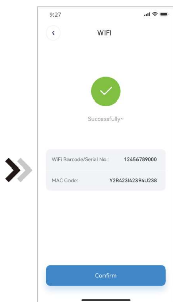
Fig.13 Enhetsbindning klart-gränssnitt
