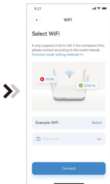
Fig.10 Ange lösenord-gränssnitt
