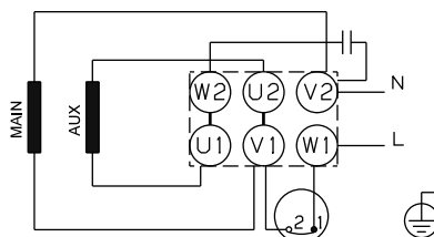
Fig. 14 Connexion, 220-230 V, 1,1 - 2,2 kW
