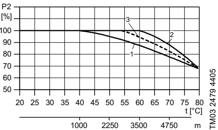
Fig. 19 Puissance moteur par rapport à la température et l'altitude
