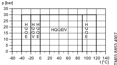
Fig. 20 Pression de service maximum admissible et température du liquide
