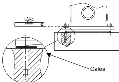
Fig. 6 Alignement avec cales
