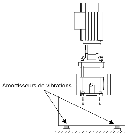
Fig. 7 Pompe sur amortisseurs de vibrations
