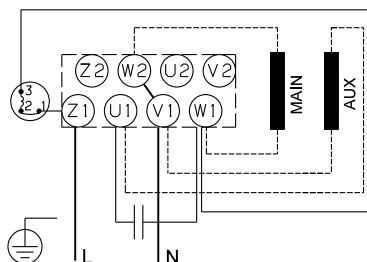
Fig. 12 Connexion, 220-230 V, 0,37 - 0,75 kW
