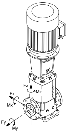
Fig. 9 Forces de bridage et couples
