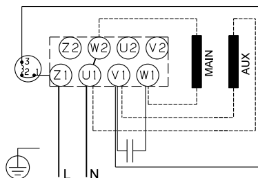
Fig. 13 Connexion, 240 V, 0,37 - 0,75 kW
