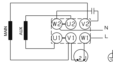
Fig. 15 Connexion, 240 V, 1,1 - 2,2 kW
