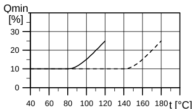
Fig. 22 Débit mini
