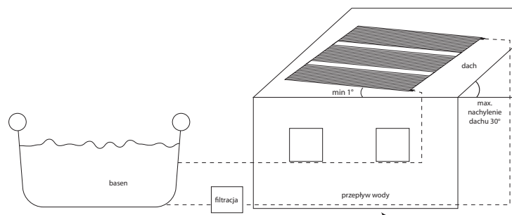
Połączenie A z blokadą przepływu
